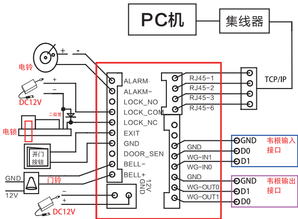
(2) 普通电源接线图
